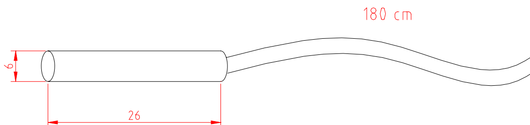
Obr. 4 Teplotní čidlo ADEX C
