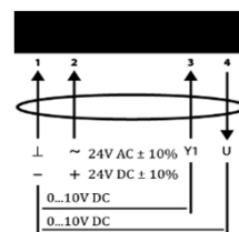
Электрическое подключение
