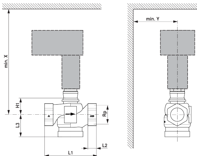
Rozměrové schéma
