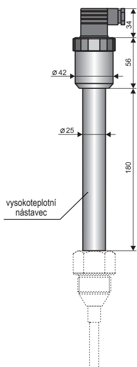
vysokoteplotní provedení CLM-36_T
