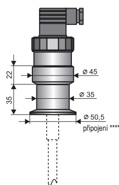
Procesní připojení Tri-clamp
