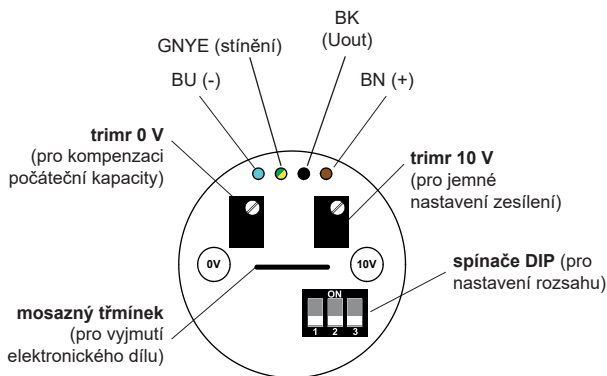
Obr. 11: Pohled shora na vnitřní elektronický díl hladinoměru s napětovým výstupem (varianta –U)
